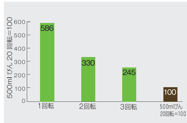
■CO 2 排出量比較(回転数シミュレーション)
